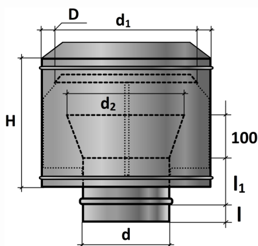
Obr. č. 11 CAGI- samotáhová hlavica
